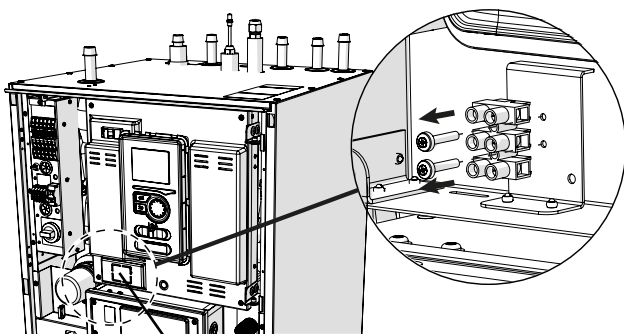
Eemaldatavad plaadid
